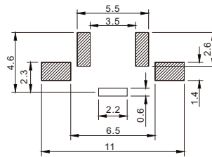
安装图 instructions
