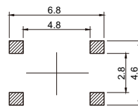
安装图 instructions
