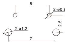
安装图 instructions
