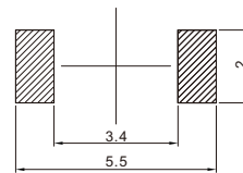
安装图 instructions
