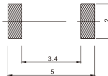
安装图 instructions
