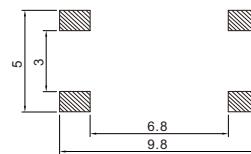
安装图 instructions
