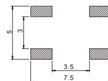
安装图 instructions
