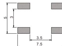
安装图 instructions
