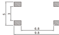
安装图 instructions
