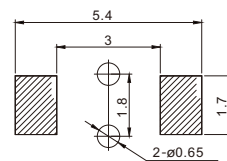
安装图 instructions
