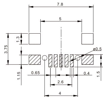
安装图 instructions
