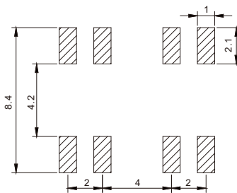
安装图 instructions
