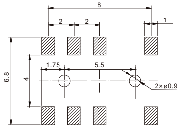
安装图 instructions
