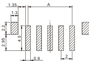
焊接图 Welding diagram
