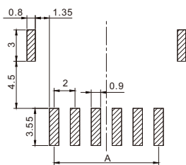
焊接图 Welding diagram
