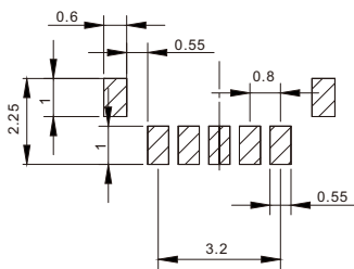
焊接图 Welding diagram
