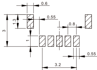
焊接图 Welding diagram
