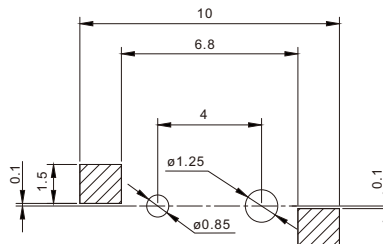
安装图 instructions
