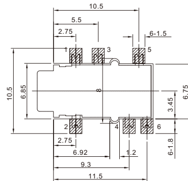
安装图 instructions
