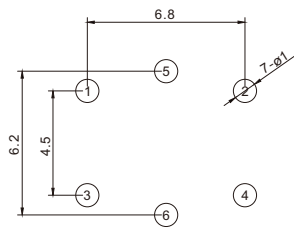
安装图 instructions
