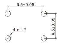
安装图 instructions
