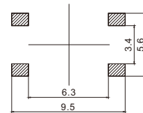
安装图 instructions
