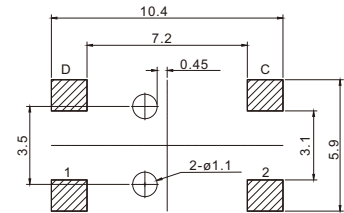
安装图 instructions
