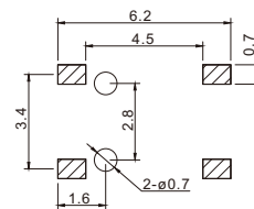
安装图 instructions
