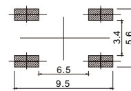
安装图 instructions
